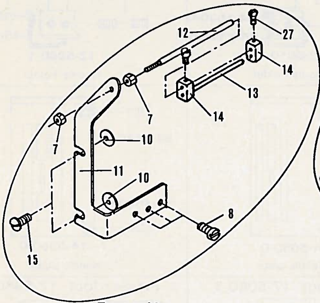
Tape guide
